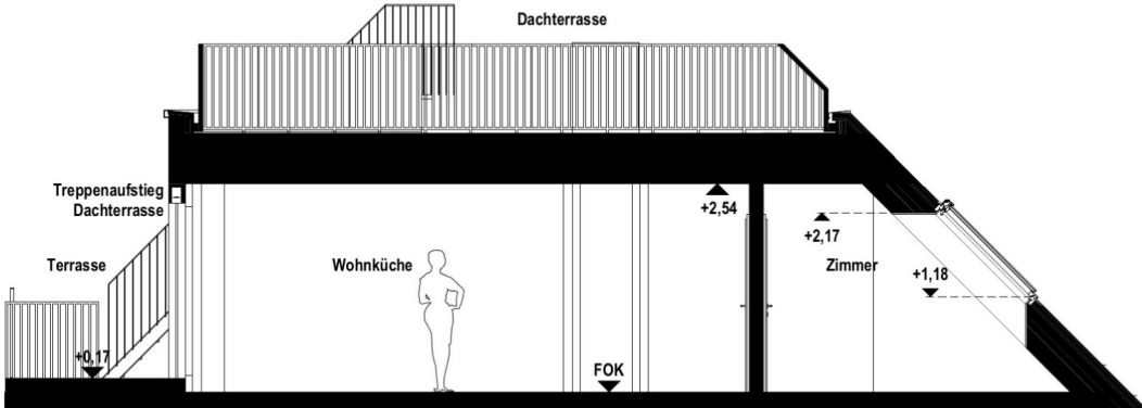
Schnitt
