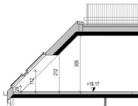
Schnitt 31.A
