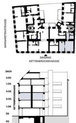
TOP 18 STIEGE 2 2. OBERGESCHOSS 2 ZIMMER Wohnung ca. 47.25m 2
