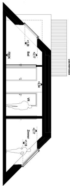
Schnitt
